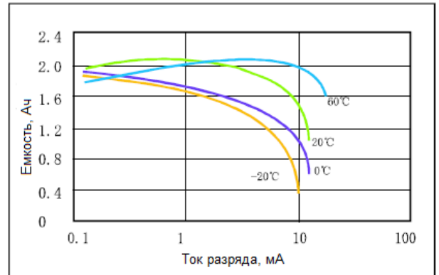
Емкость при различном токе разряда
