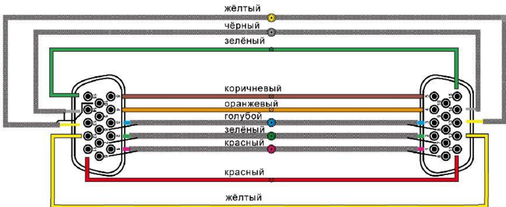
Схема распайки кабеля:
