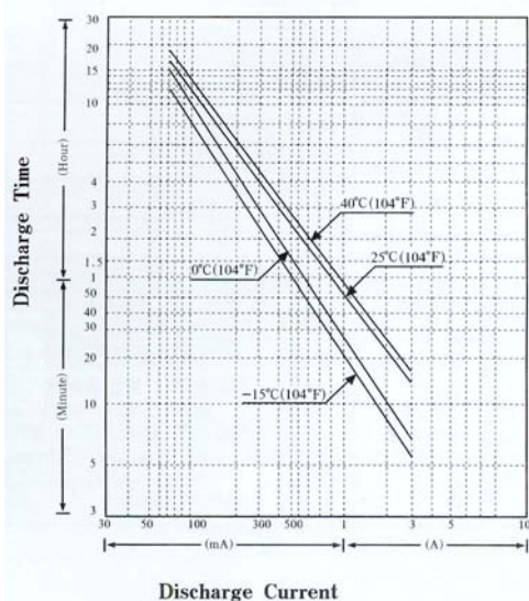
Ток разряда от времени разряда.
