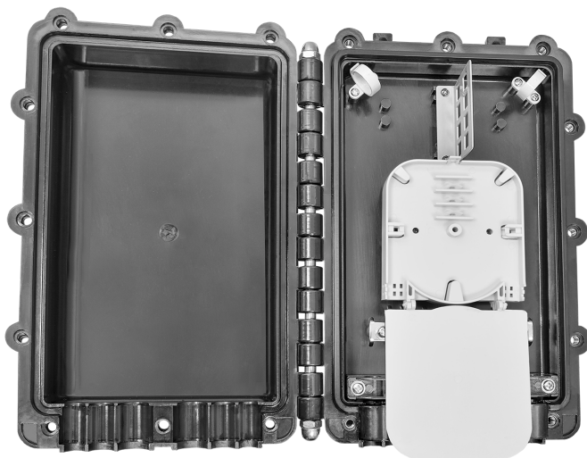
Рисунок 2 - Внутренний конструктив
