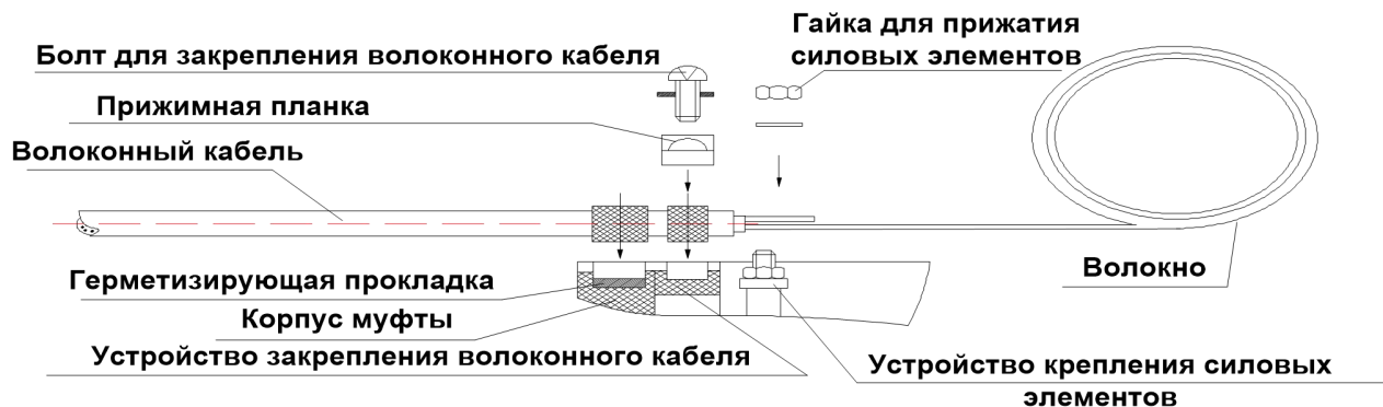
Рисунок 5 - Закрепление силовых элементов и волоконного кабеля
