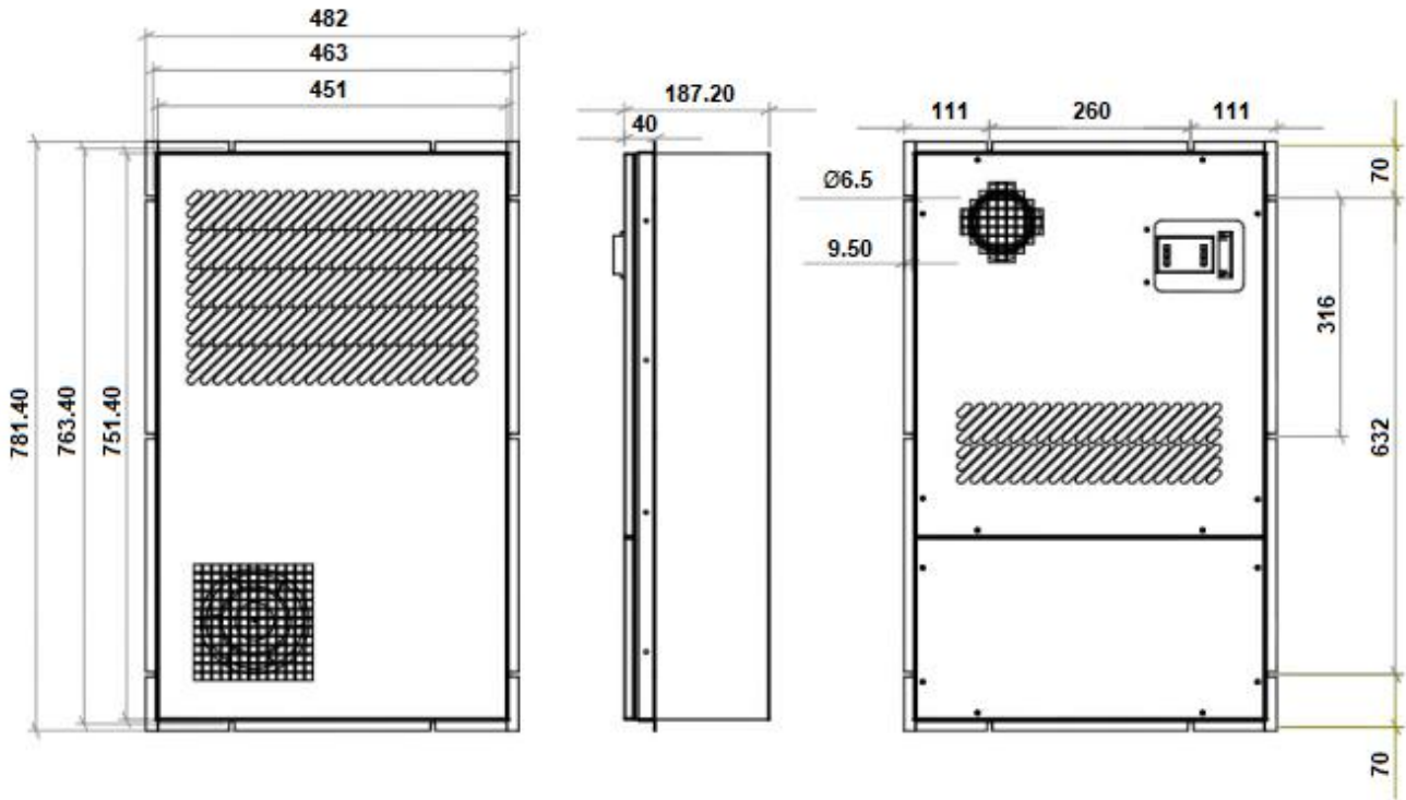
Рисунок 6 Габаритные размеры SNR-ACC-1500
